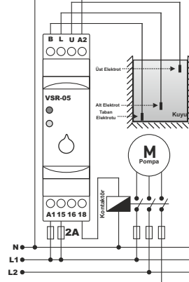
VSR-05 için bağlantı şeması
