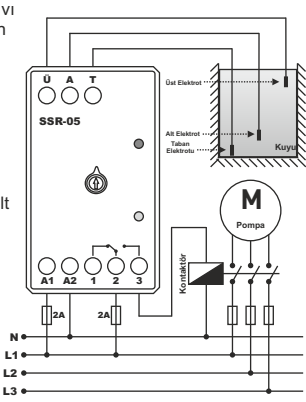
SSR-05 için bağlantı şeması
